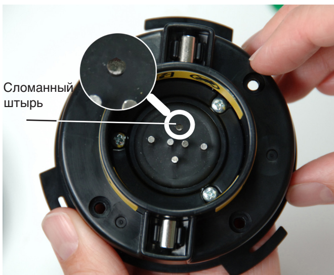
Рисунок 5 – Сломанный контактный штырь
